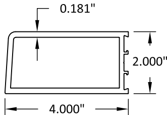
⑩④ HINGE STILE
