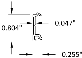
⑤ DOOR SWEEP BASE (OPTIONAL)
