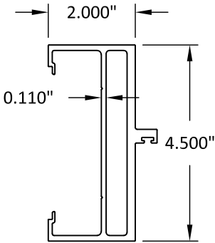
② DOOR JAMB O/P
